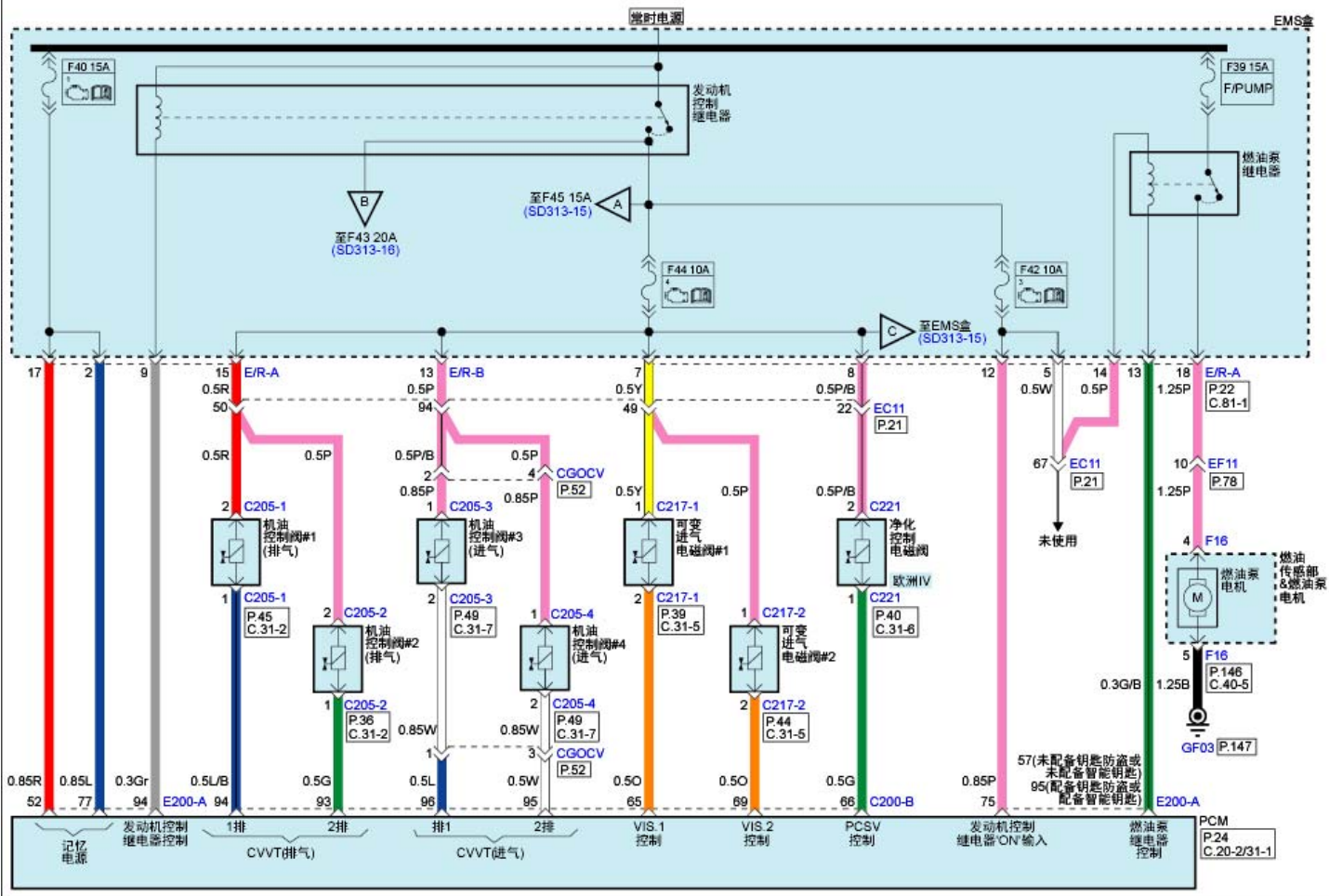
发动机控制系统(G6DG/G6DH : LAMBDA-II 3.0L/3.3L GDI)(5)
